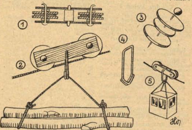
Seilbahn aus Pappendeckel. 1 = Lautwerk im Querschnitt, 2 = Holztransport, 3 = 3 Pappendeckelscheiben werden zu einem Lauftrad zusammengeklebt, 4 = Aufhängevorrichtung, 5 = Seilbahnwagen.
