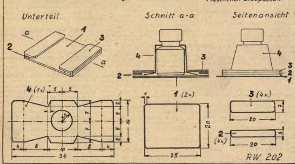
Fig. 1 Ständer für Tuschfläschchen. Die Maße sind dem eigenen Fläschchen anzupassen.
